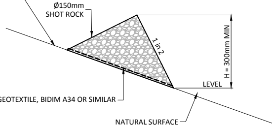
ELEVATION 1 N.T.S
