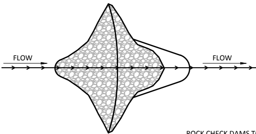
PLAN N.T.S
