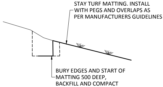
STAY TURF EDGE DETAIL N.T.S.
