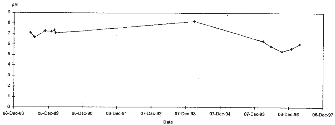
GBMB3 - pH
